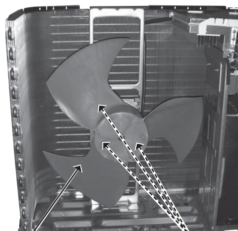
Propulsor Tornillos del motor del ventilador exterior
